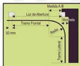
Art. 12 | 21 Perfil para Guía U
